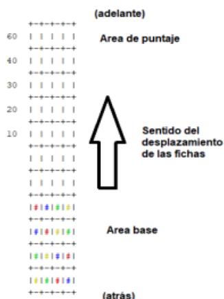
Fig. 1 Juego "Saltar"
