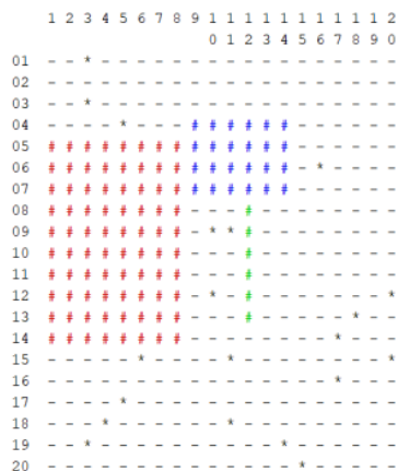
Fig. 2 Juego "Rectángulo"
