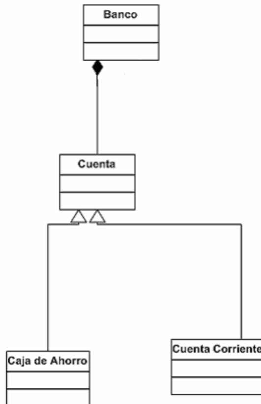
Ilustración 17 Banco
