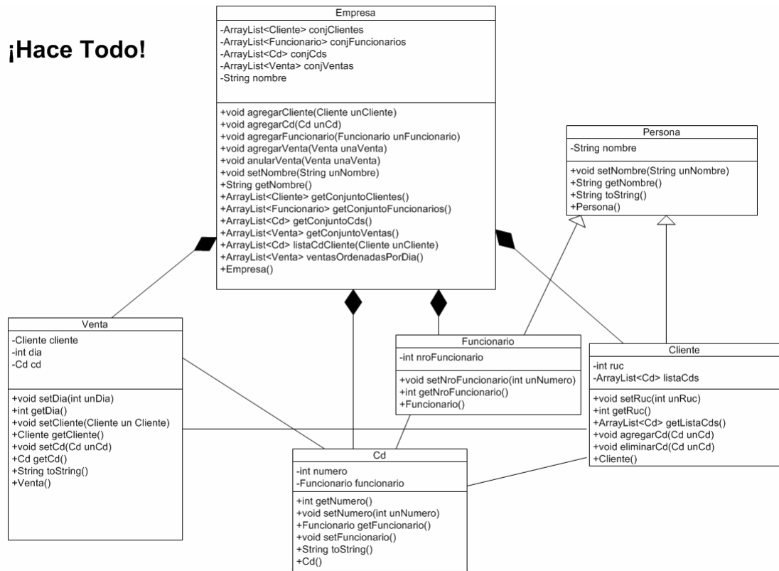
Ilustración 20 HaceTodo
