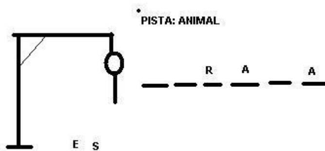
Ilustración 3 Ahorcado
