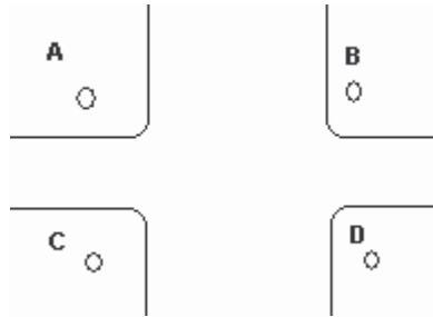
Ilustración 2 Semáforo
