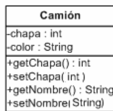
Ilustración 11 Clase Camión
