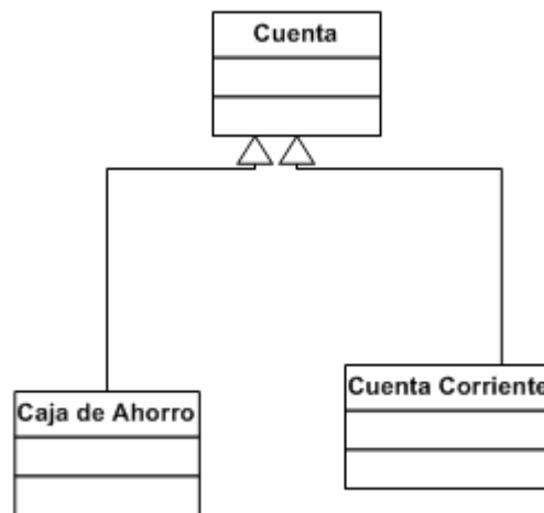
Ilustración 16 Cuenta
